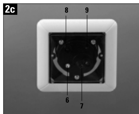
Fig. 2a 1 Telaio frontale 2 Copertura frontale lente Fig. 2b 3 Jumper campo di misura 4 Morsetto 5 Jumper detettore/interruttore bistabile Fig. 2c 6 Pot. regolazione del campo di misura 7 Trasmettitore 8 Ricevitore 9 LED rosso, indicazione di funzione
